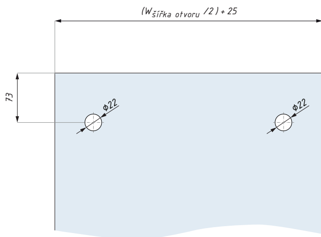
Příprava skla, fixní panel Glass preparation, fixed panel
