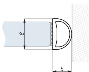
montáž na zed' wall installation
